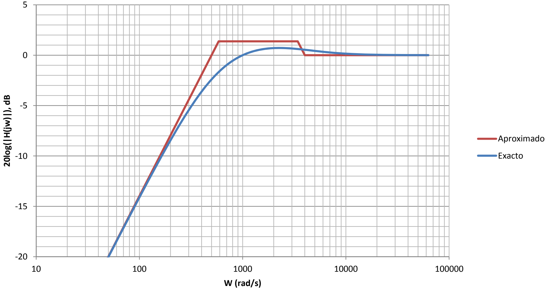
Módulo de Bode (polos y ceros del problema)
