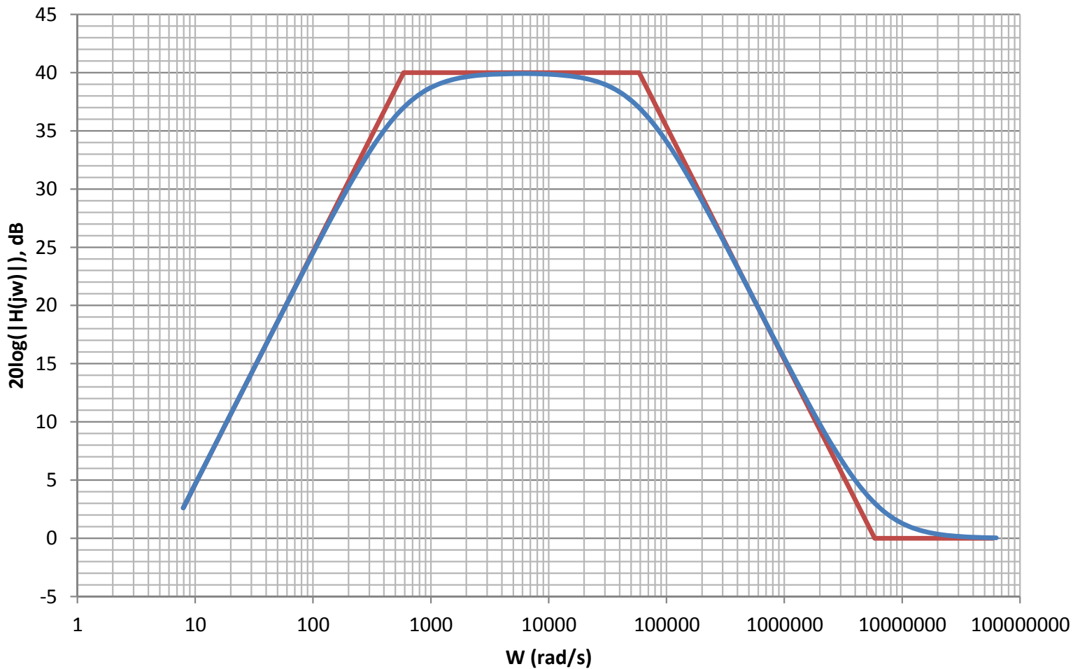
Módulo de Bode (polos y ceros alejados)
